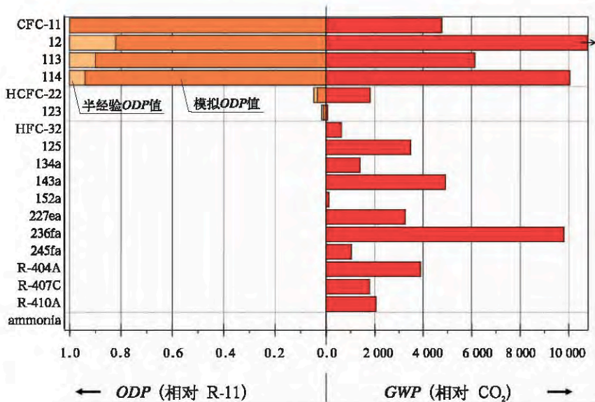
图 2 主要制冷剂的臭氧损耗潜能值(ODP)与全球温室效应潜能值(GWP)对比
